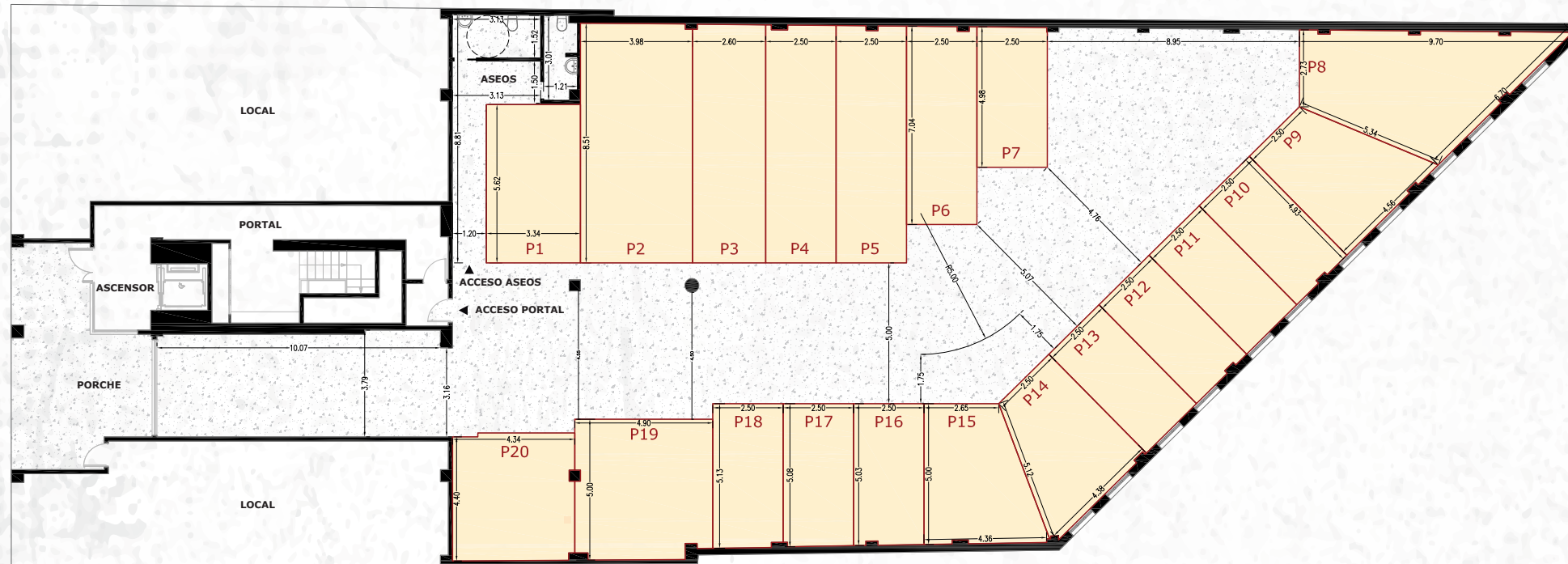
PLANTA BAJA
